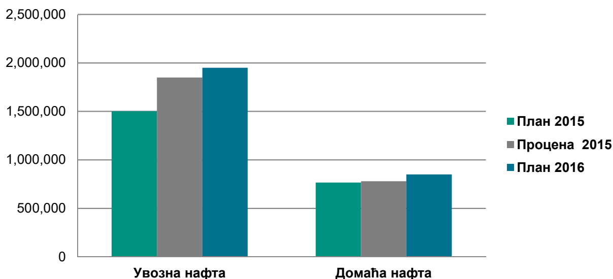
График 2 План транспорта за 2016. годину по пореклу нафте упоредо са планом и проценом за 2015. годину
